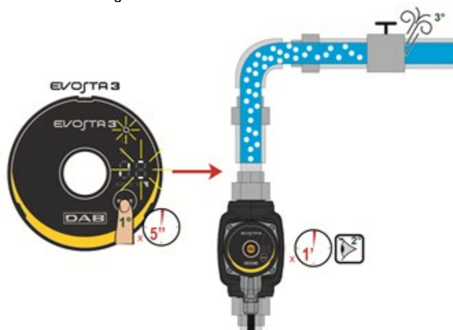
Abb. 9: Automatische Pumpenentlüftung
