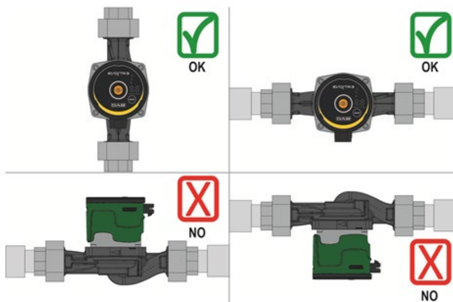
Obrázok 3: Montážna poloha
