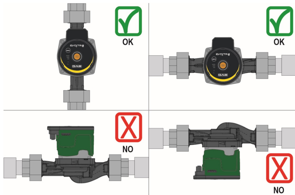
Εικόνα 13: Θέση συναρμολόγησης
